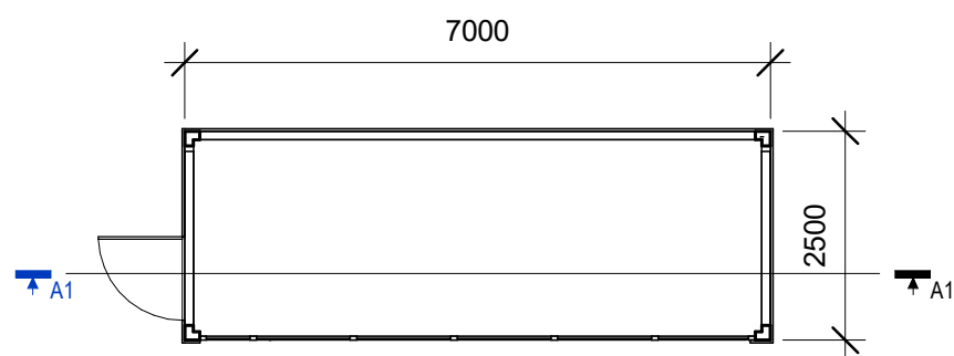
Kiosko planas 1 : 100
