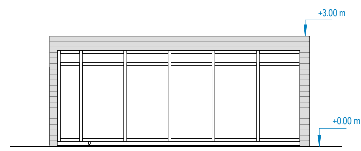
Kiosko fasadas 1 : 100
