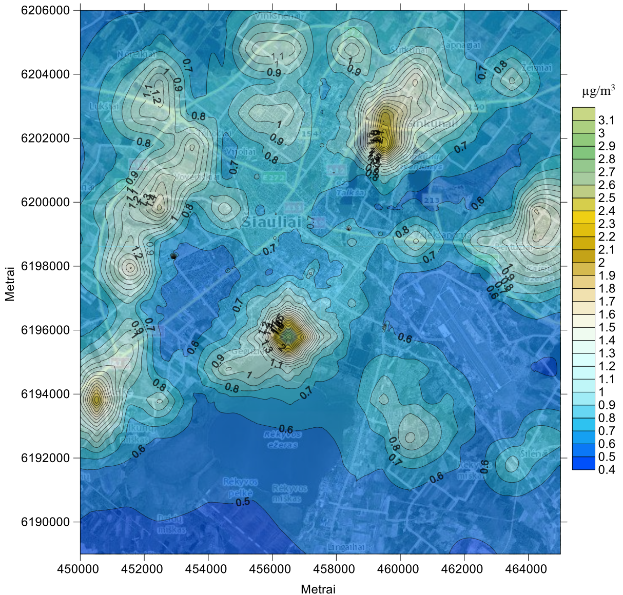
1.31 pav. Sieros (II) oksido 24 valandos 99.2 procentilio koncentracija aplinkos ore
