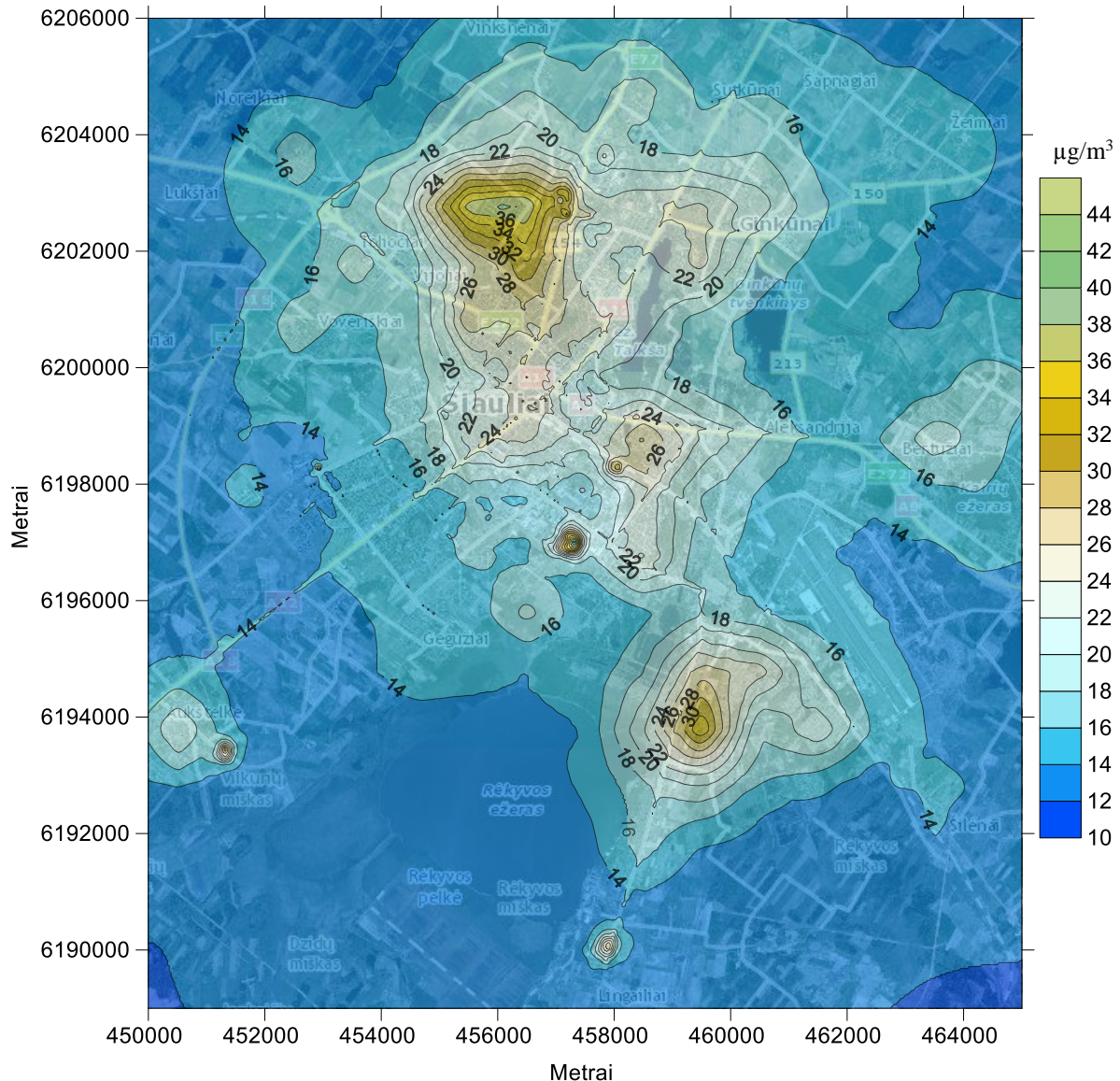
1.29 pav. Kietosios dalelės ( \text{KD}_{10} ) 24 valandų (paros) 90,4 procentilio koncentracija aplinkos ore
