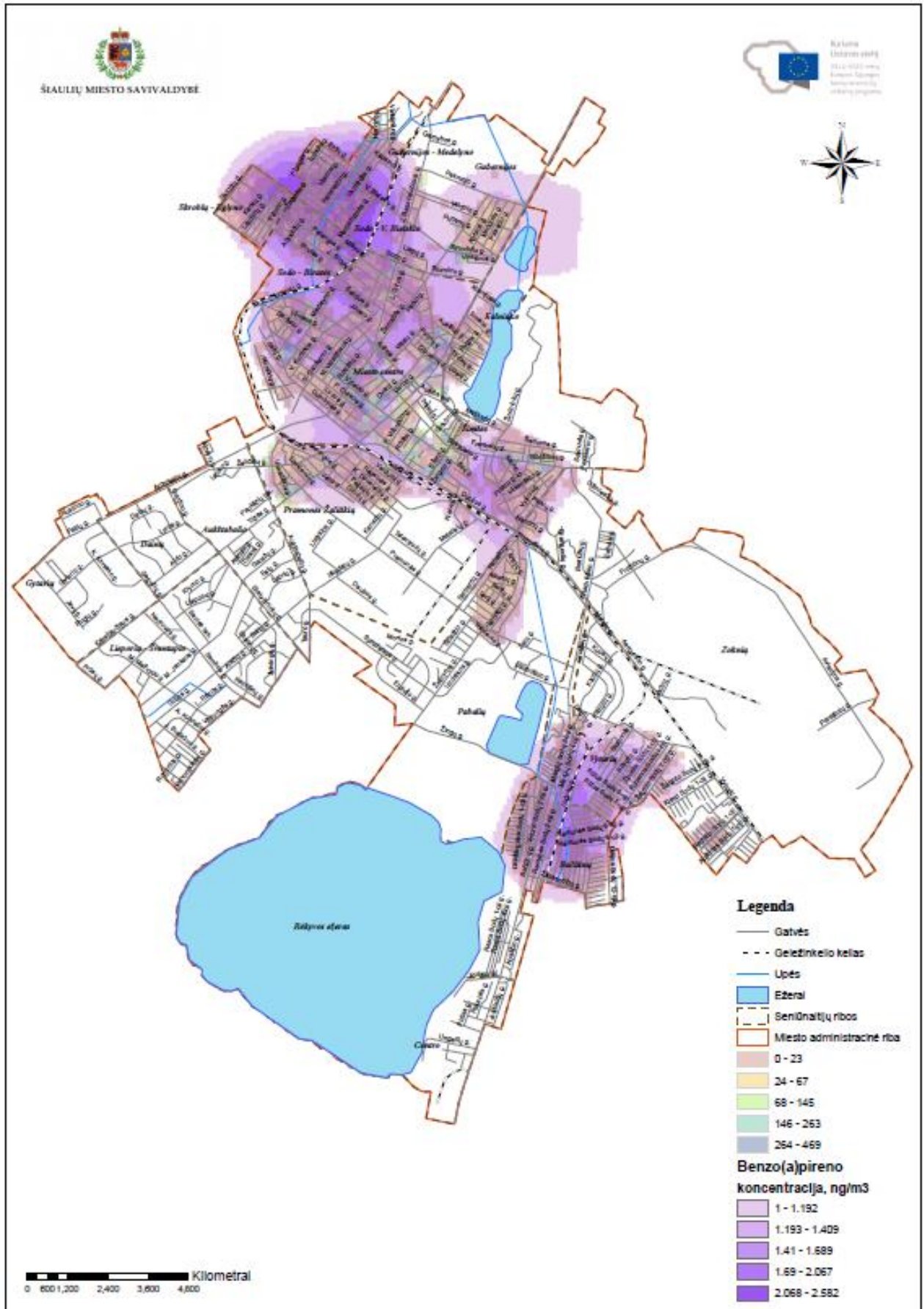
3.3 pav. Aplinkos oro taršos benzo(a)pirenu viršijimo teritorijos aprėptis Šiauliuose mieste
