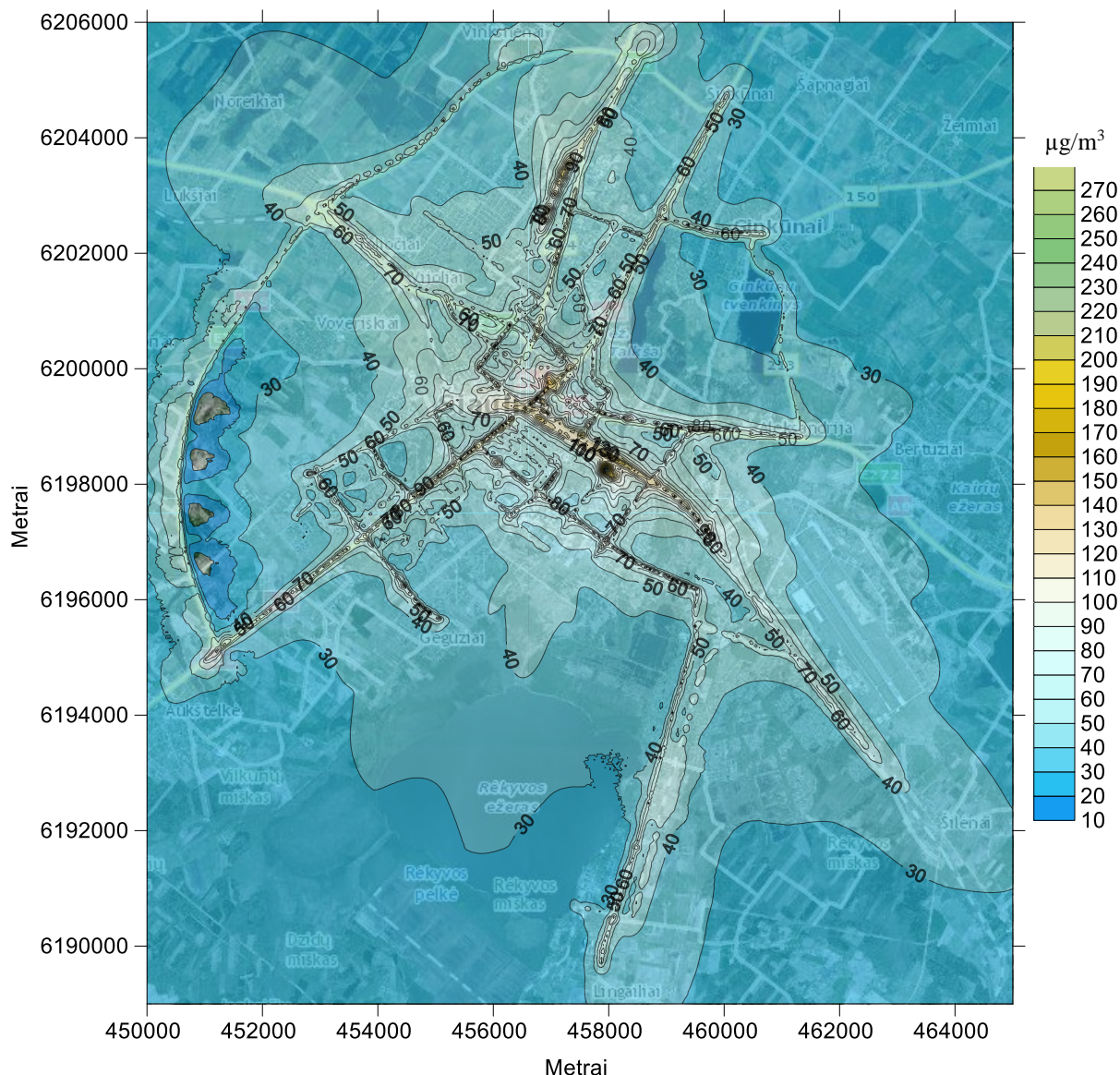
1.28 pav. Azoto (II) oksido 1 valandos 99.8 procentilio koncentracija aplinkos ore
