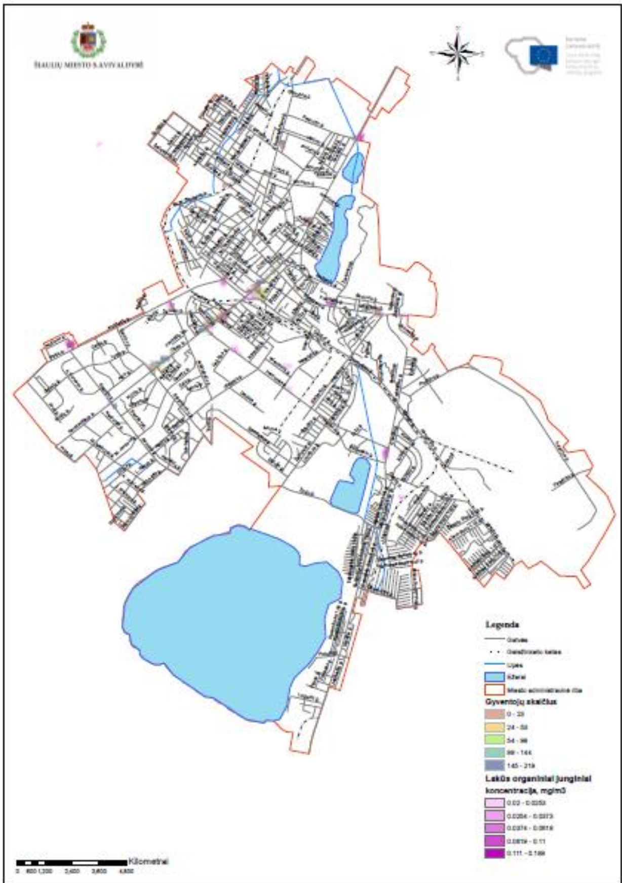
3.8 pav. Lakiųjų organinių junginių sklaidos aprėptis, vertinant aukštesnę taršos lygį nei 2 % ribinės vertės
