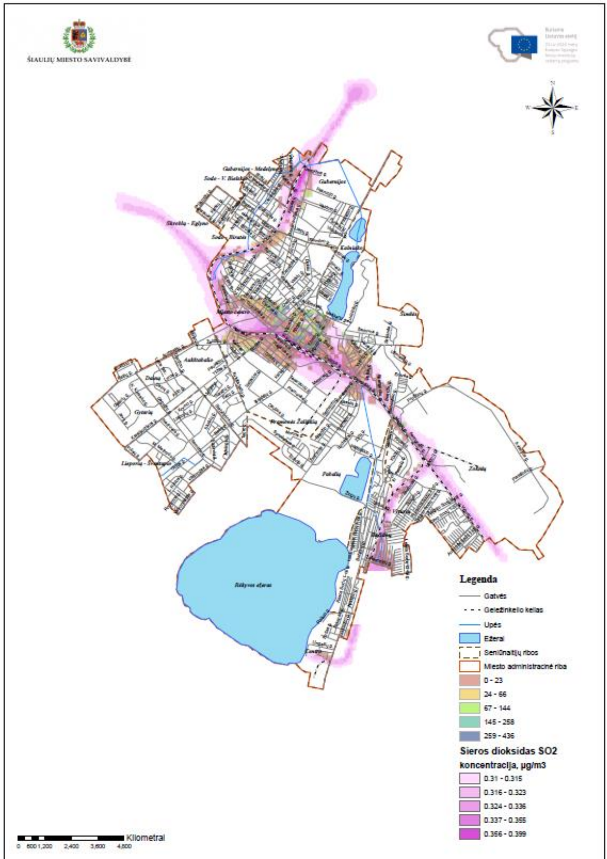
3.9 pav. Geležinkelio transporto sieros dioksido sklaidos aprėptis, vertinant aukštesnį taršos lygį nei 0,24 % ribinės vertės
