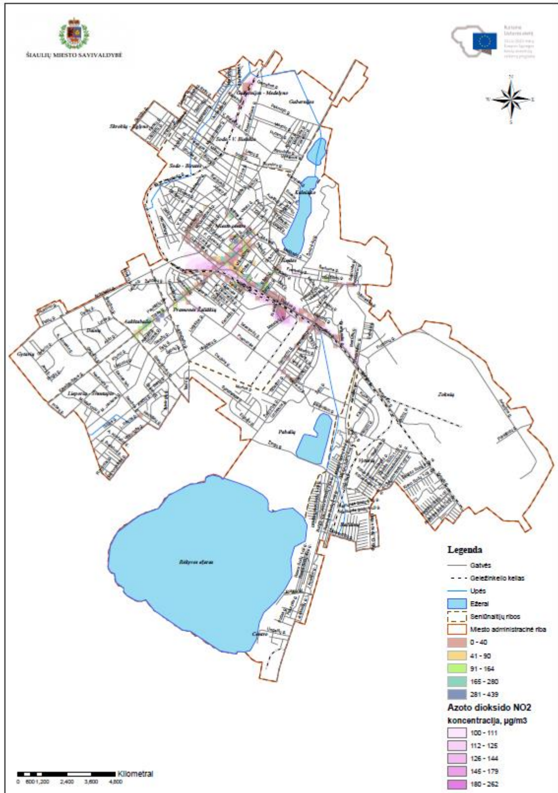
3.6 pav. Azoto dioksido NO 2 sklaidos aprėptis, vertinant aukštesnį taršos lygį nei 50 % ribinės vertės
