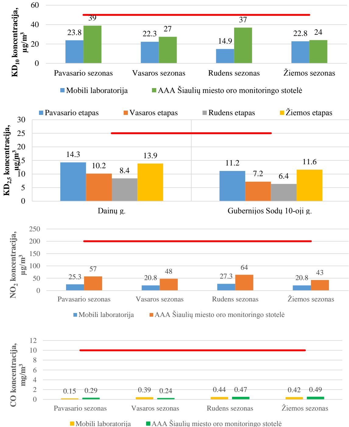
1.26 pav. Šiaulių mieste skirtingais sezonais (pavasario, vasaros, rudens ir žiemos) išmatuotos kietųjų dalelių, anglies monoksido ir azoto dioksido koncentracijos (raudona linija – ribinė vertė)
