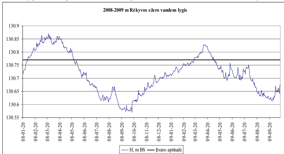
1 pav. 2008-2009 m. Rėkyvos ežero vandens lygis
